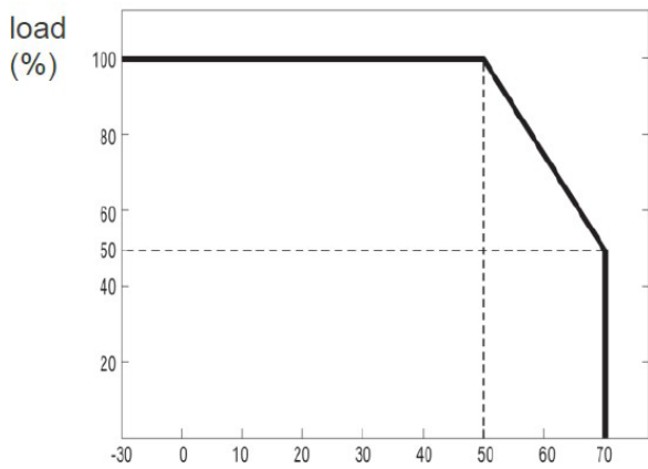
Environment temperature(°C)
